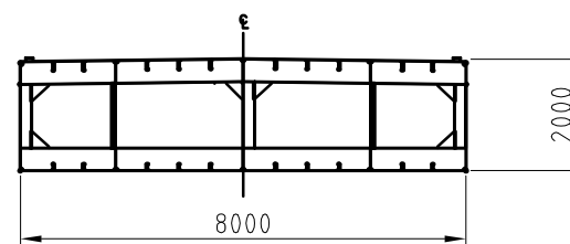
WEB FRAME (spacing 2400mm)
