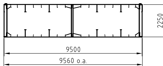
NormalFrame (spacing 600mm)
